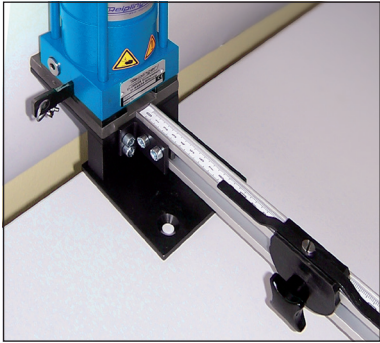
Poinçonnage pneumatique trou Ø 10,1 mm et découpe des tringles de traction.
