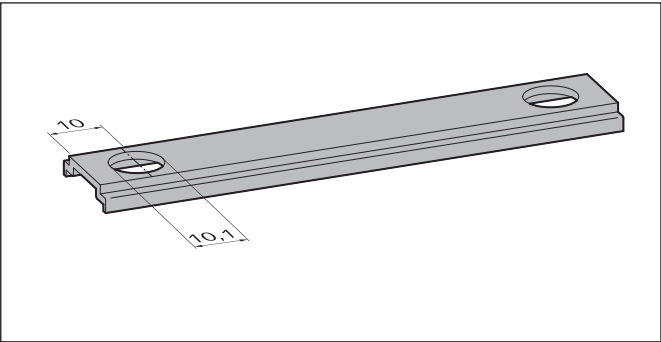
Perçage d'un diamètre de 10,1 mm
