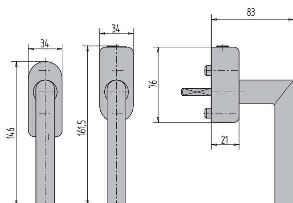
Positionnement du cylindre haut Positionnement du cylindre bas
