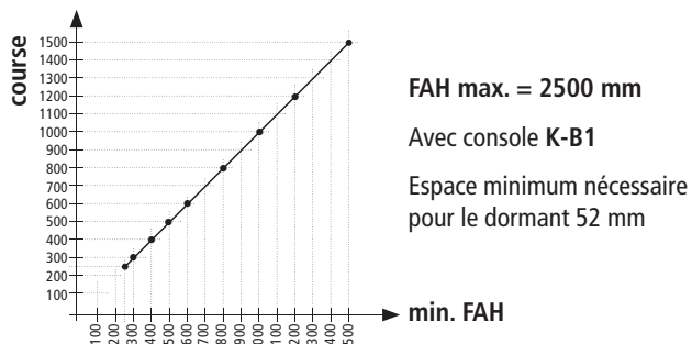
Châssis abattant
