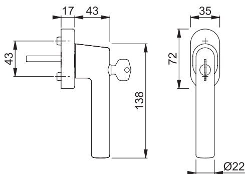
Poignée de fenêtre Hoppe Amsterdam E0400S/US9056
