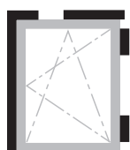
Ferrures oscillo-battantes inversées
