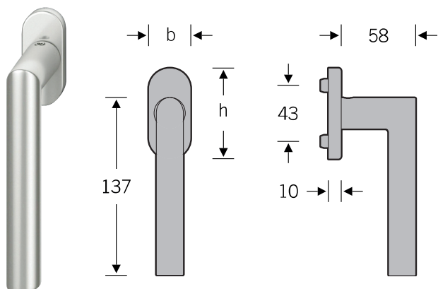
Poignée de fenêtre FSB modèle 34 1076
