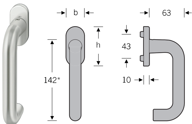
Poignée de fenêtre FSB modèle 34 1070
