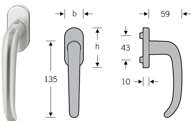
Poignée de fenêtre FSB modèle 34 1023
