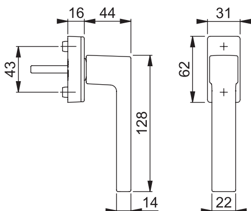
Poignée de fenêtre Hoppe Austin 0769/US947
