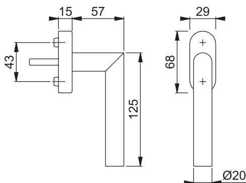
Poignée de fenêtre Hoppe Amsterdam E0400/U30
