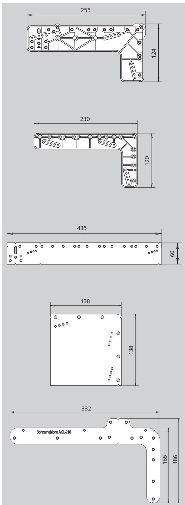
Gabarit de perçage AK-210
